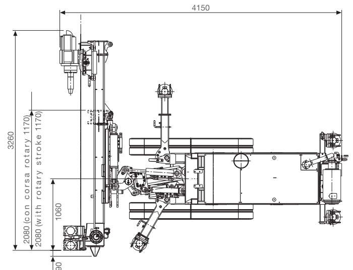
Disegno 4 / Drawing 4 Esecuzioni di tiranti / Anchor execution
