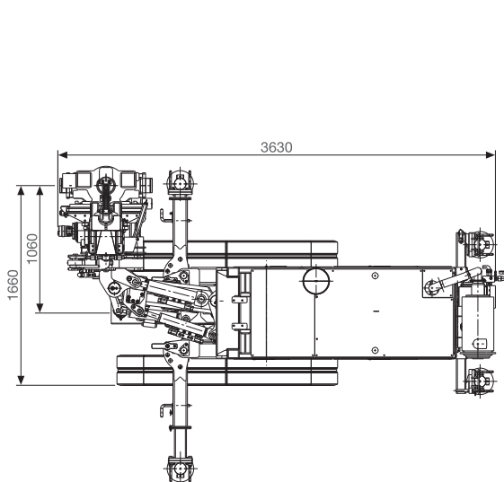
Disegno 3 / Drawing 3 Perforazioni verticali in prossimità di pareti / Drilling near vertical walls
